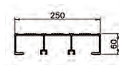
Golvprofil
